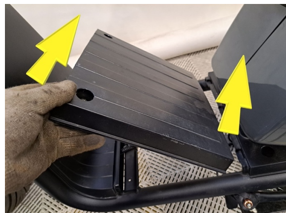
Ota jalkatilan päällyskate pois.
