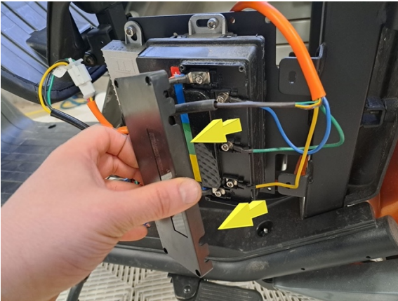
Ota ohjainlaitteen suojakansi pois.
