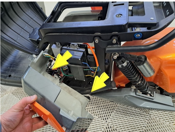
Ota vasen kylkipaneeli pois.
