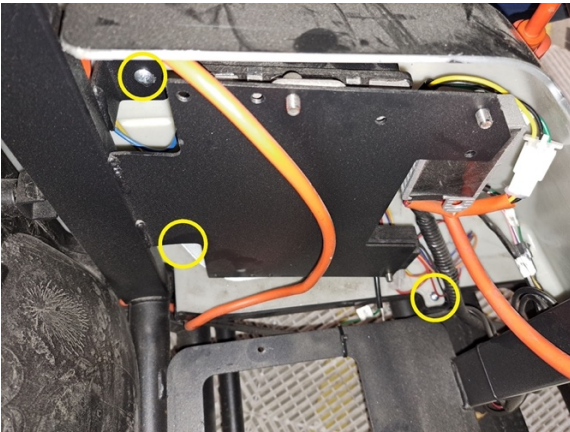
Irrota vasemman kylkipaneelin kolme kiinnitysruuvia. (ristipäämeisseli).
