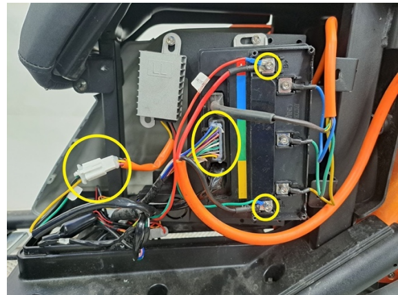
Avaa muuntajan liitin. Irrota ohjainlaitteen liitin. Irrota ohjainlaitteen- ja + johdot. (kuusiokoloavain 4 mm).
