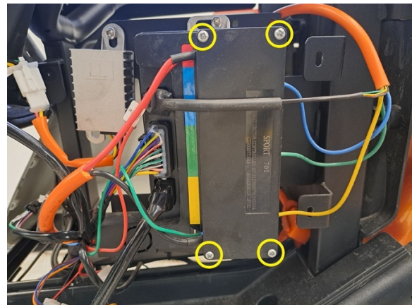
Irrota ohjainlaitteen suojakannen neljä kiinnitysruuvia. (ristipäämeisseli ph2).
